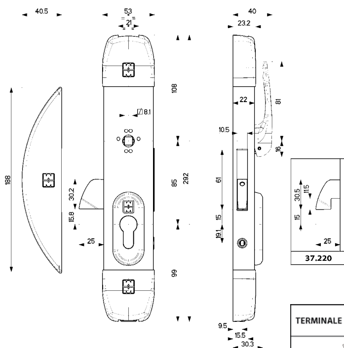
CHIAVISTELLO PIATTO
