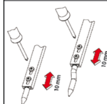
TERMINALE REGOLABILE
